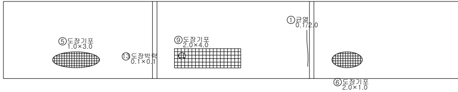
배면벽체
